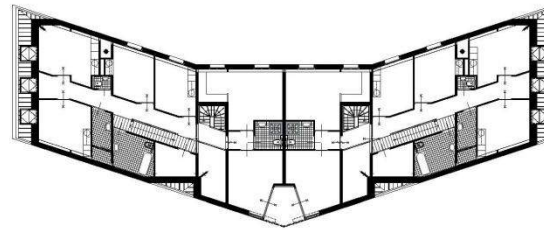
verdieping
