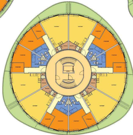
kopappartementen / villa 4
