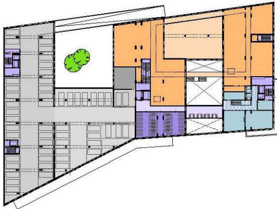
1e VERDIEPING
