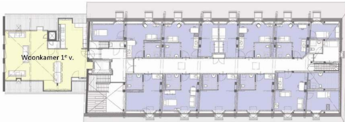
1° verdieping
