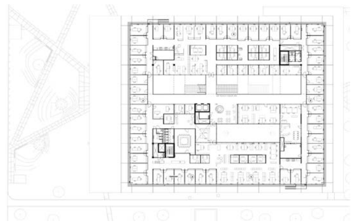
Plattegrond - tweede verdieping
