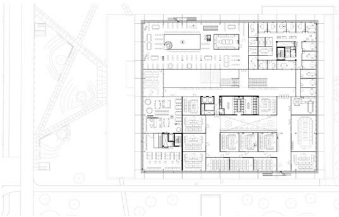
Plattegrond - eerste verdieping
