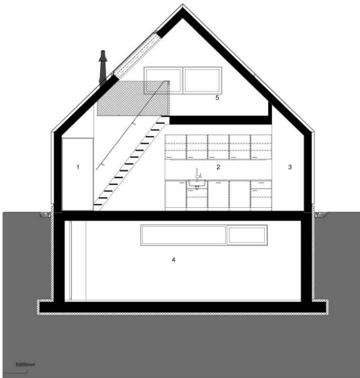
Doorsnede voorzijde
