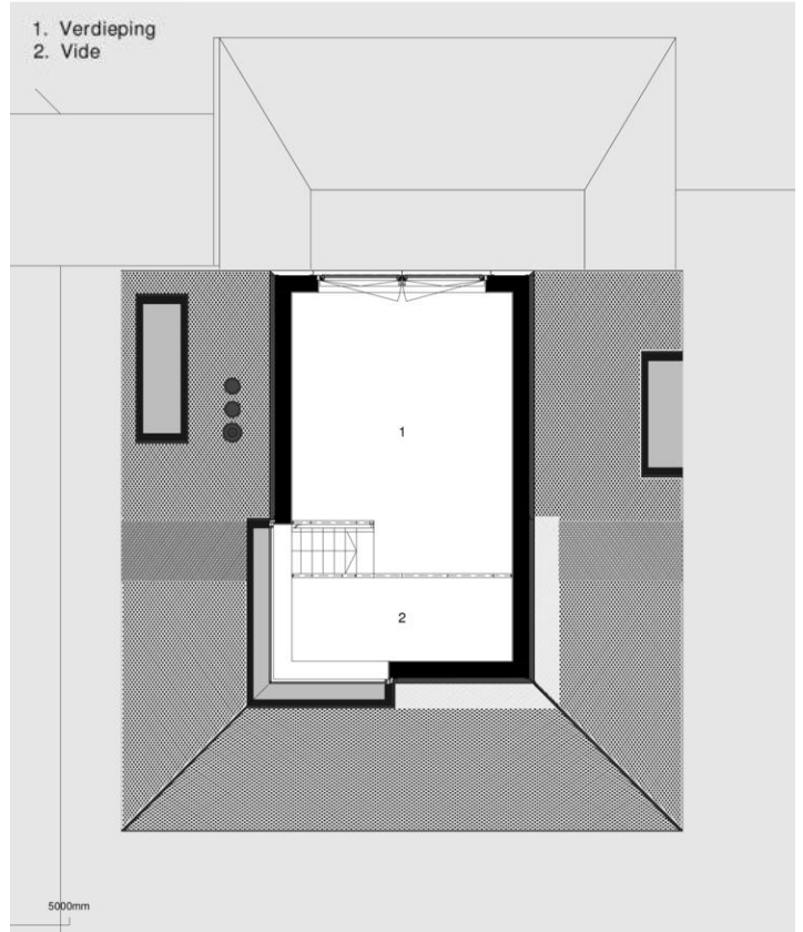
Plattegrond eerste verdieping
