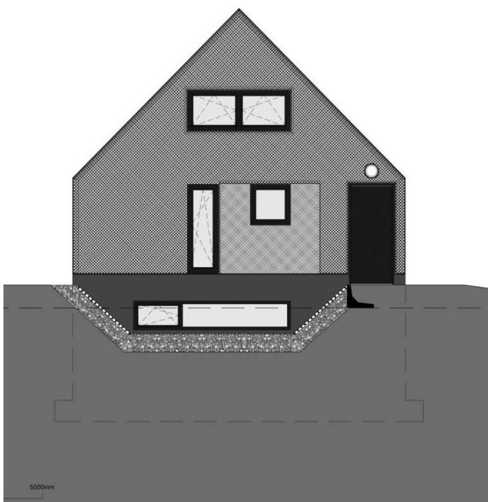
Gevelaanzicht achterzijde
