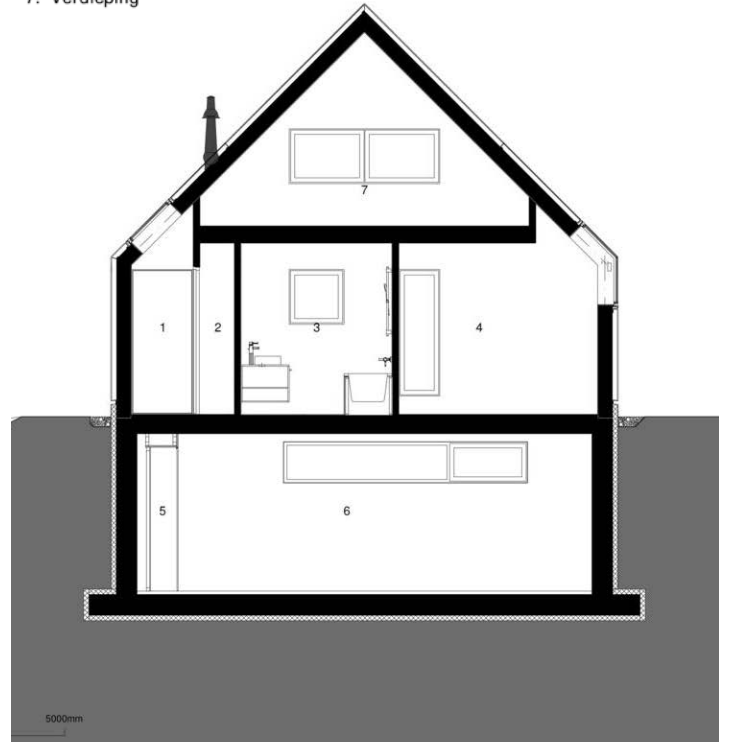
Doorsnede achterzijde
