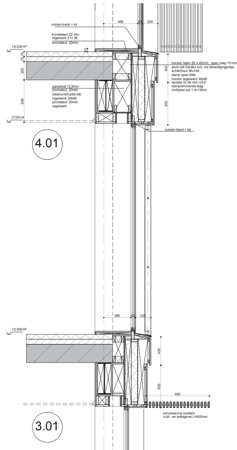
geveldoorsnede verticaal
