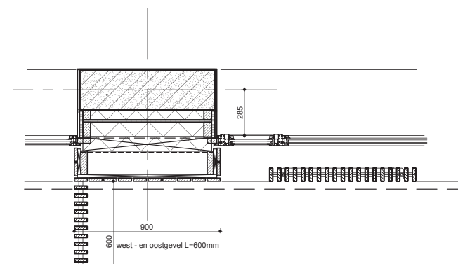
geveldoorsnede horizontaal
