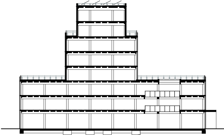
Doorsnede
