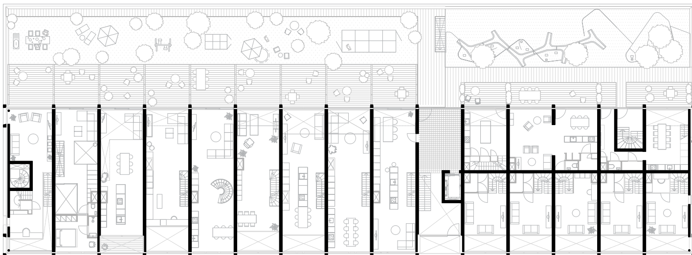
Plattegrond laag 01
