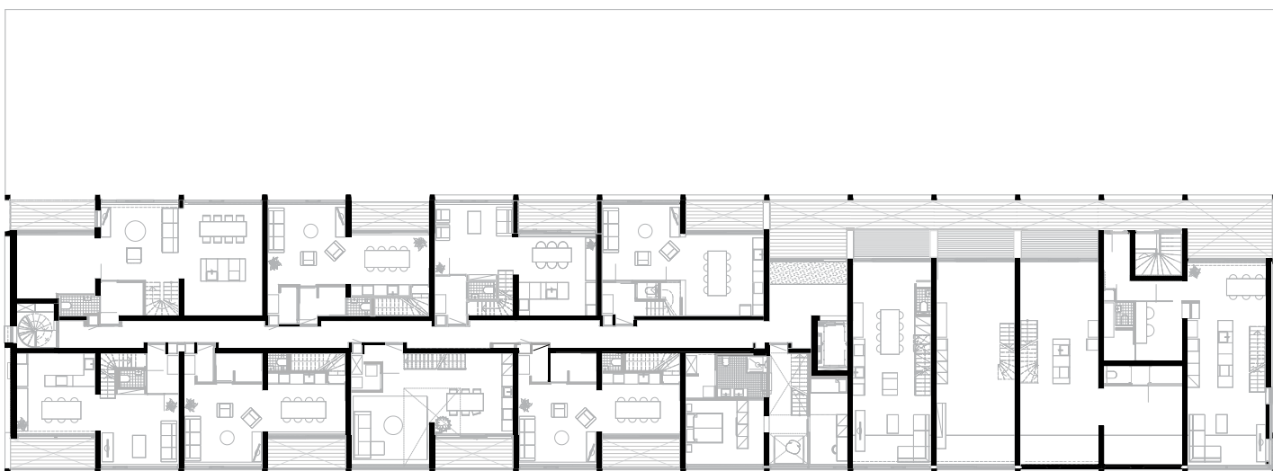
Plattegrond laag 03
