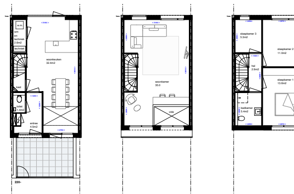
Type A2 Extra slaapkamer, Techniek en WM op begane grond
