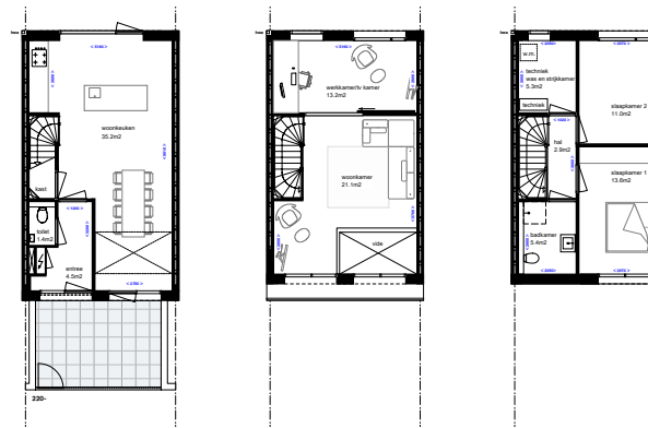
Type A3 Werk/Studeer/TV-kamer op verdieping
