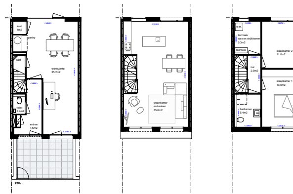
Type A1 Werkruimte op begane grond met eigen entree
