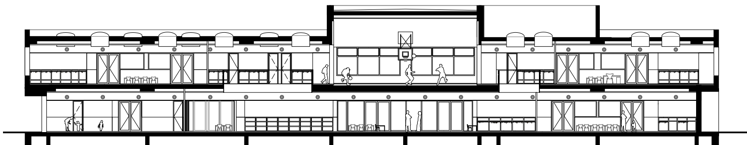
Langsdoorsnede
