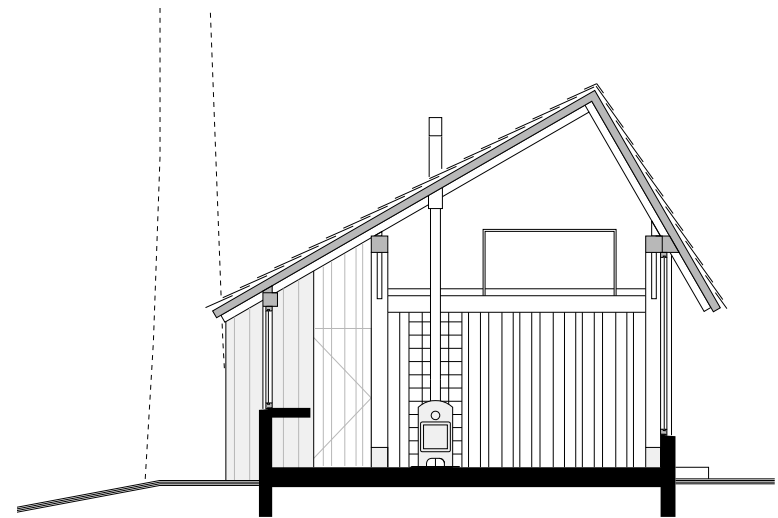
doorsnede werkplaats
