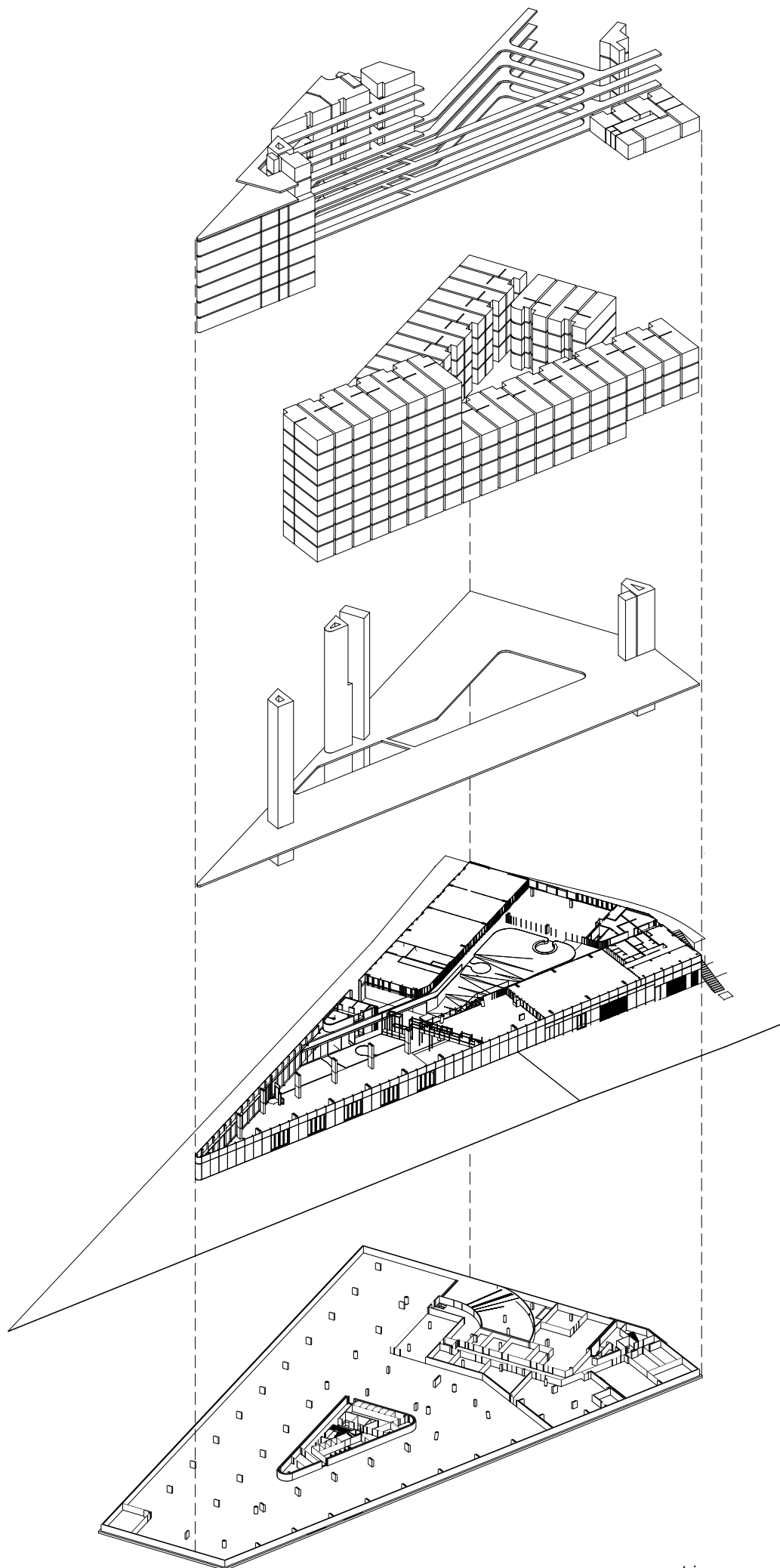
axonometrie
