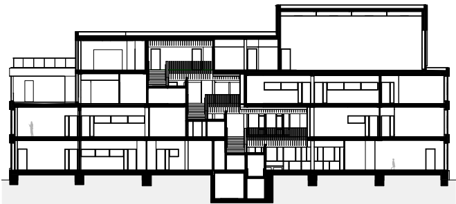
doorsnede
