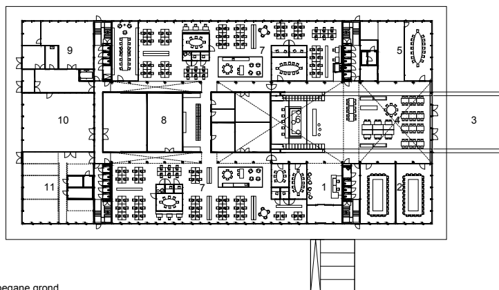
begane grond
