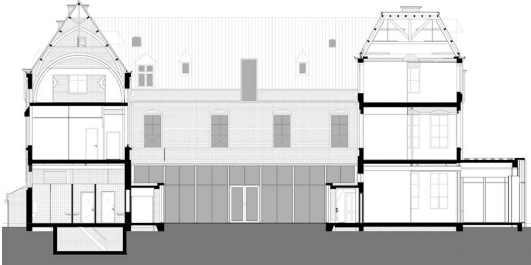
DWARSDOORSNEDE
