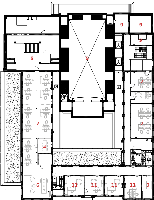
EERSTE VERDIEPING
