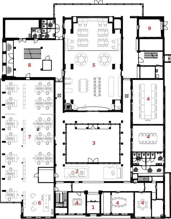
BEGANE GROND
