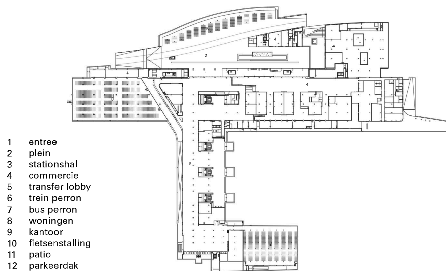
plattegrond niveau 1
