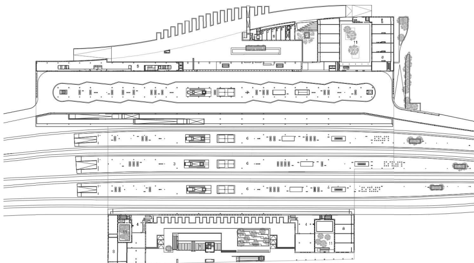
plattegrond niveau 1
