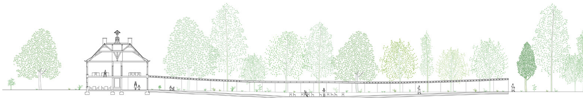
Langsdoorsnede met verdiept auditorium voor 100 personen
