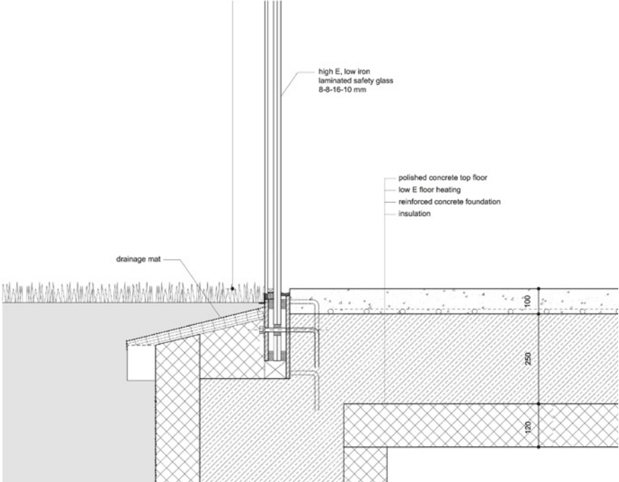
Geveldetail gang
