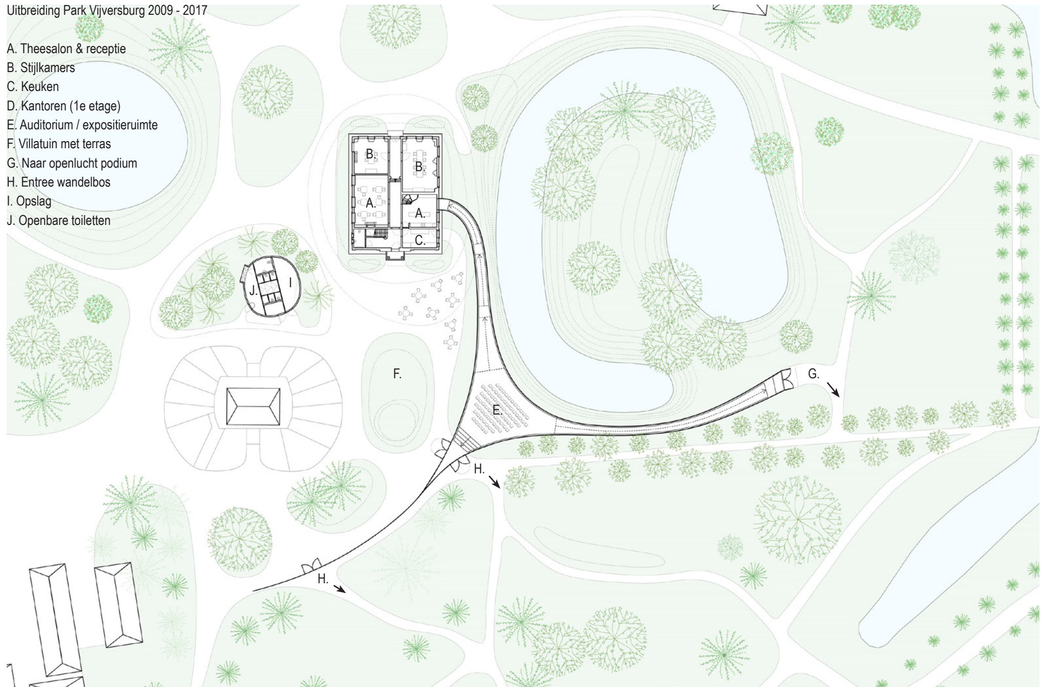
Plattegrond bezoekerscentrum
