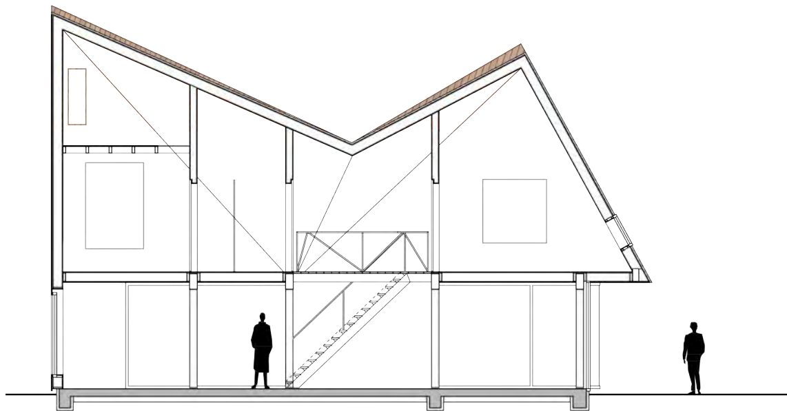
DOORSNEDE A
