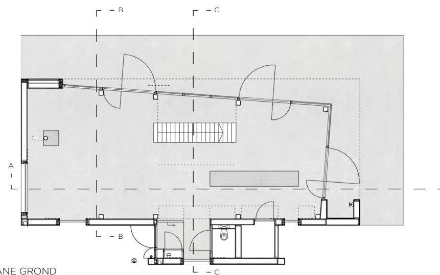
BEGANE GROND
