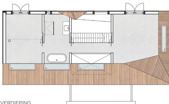
EERSTE VERDIEPING
