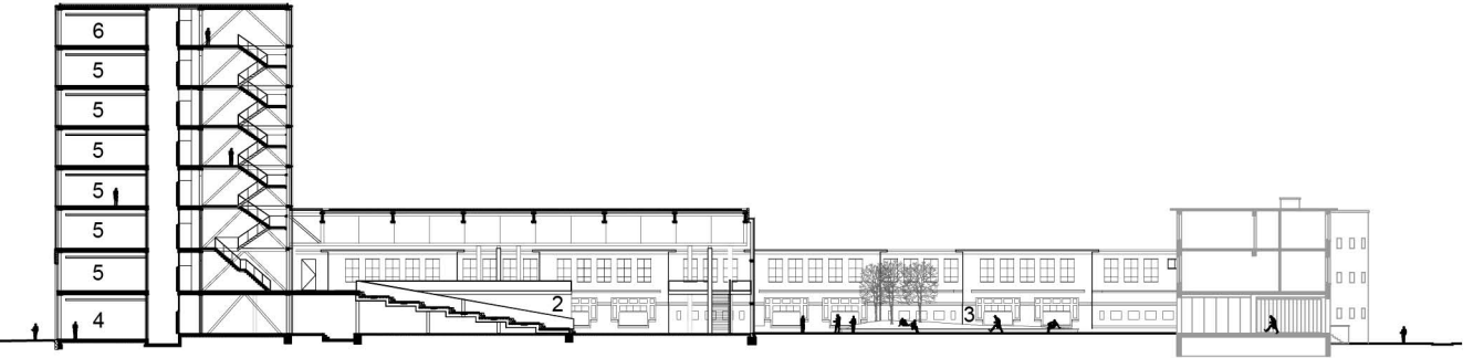
langsdoorsnede nieuwe situatie
