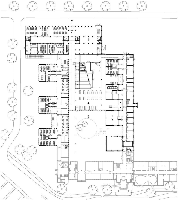
begane grond nieuwe situatie
