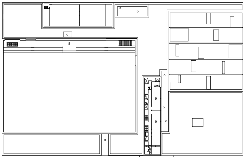
plategrond niveau 1
