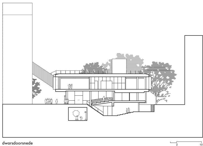
dwarsdoorsnede
