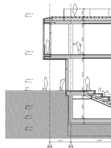
doorsnede over gevel
