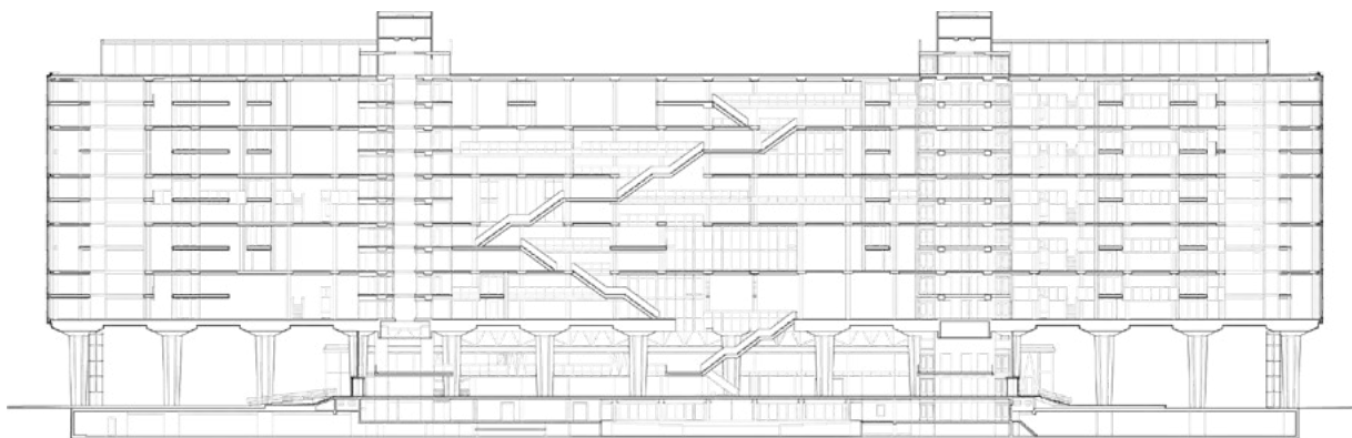
Langsdoorsnede: centrale rode trap
