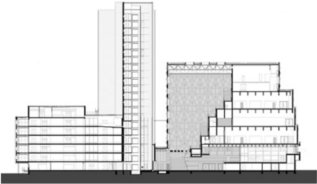
Doorsnede
