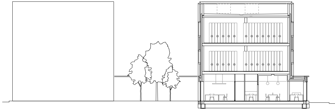
Dwarsdoorsnede
