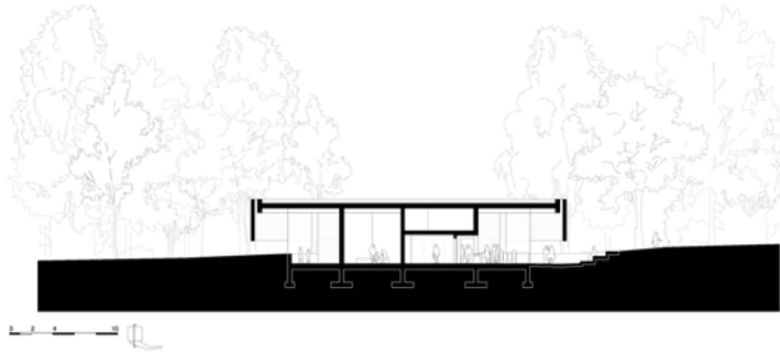
Doorsnede AA
