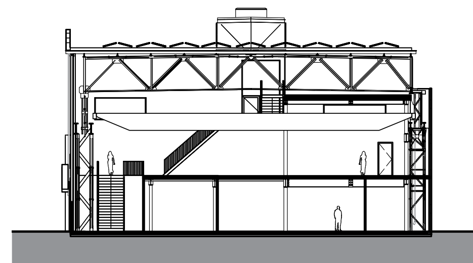
doorsnede B-B
