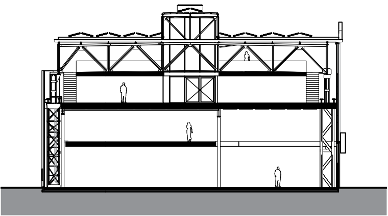
doorsnede C-C
