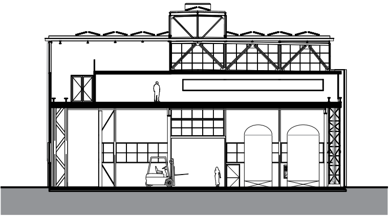
doorsnede E-E
