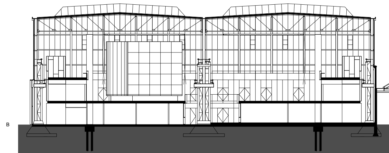
dwarsdoorsnede
