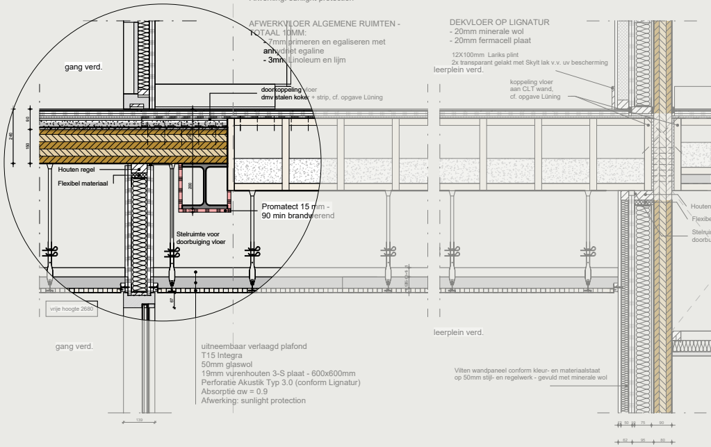
In dit detail is zichtbaar hoe de verschillende technieken elkaar aanvullen. Massieve houten en holle houten kanaalvloeren.
