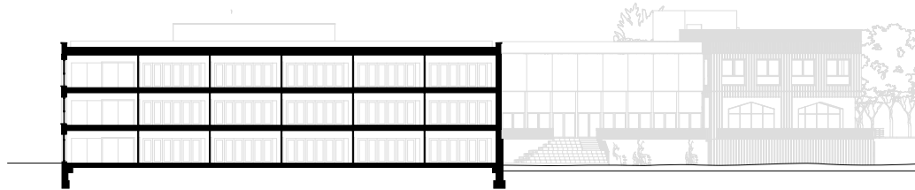
Langsdoorsnede deelschool
